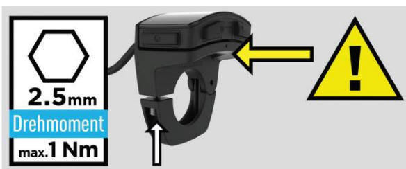
Abbildung 2: Richtiges Drehmoment, Druck auf das Gehäuse vermeiden
